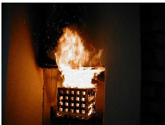
Fotografia: Teste de Incêndio em Fachada
